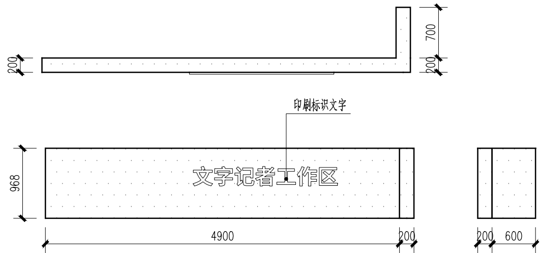
标识围挡详图
