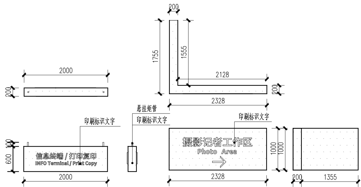
悬挂导视详图
